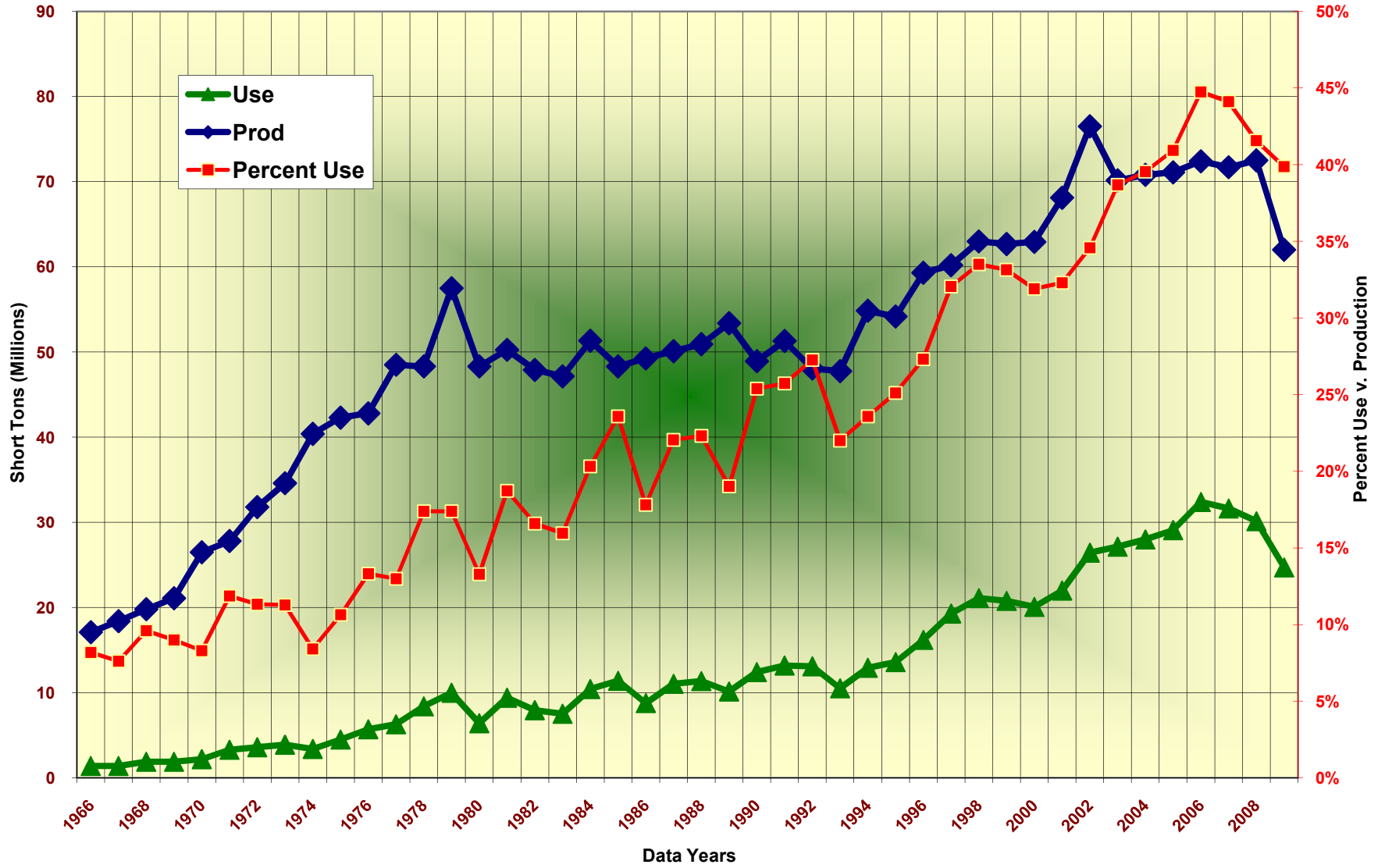
ACAA Fly Ash Production & Use Comparisons 1966-2009
